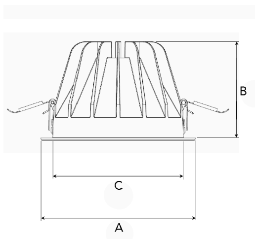
A 195 B 122 C 178 (mm)
